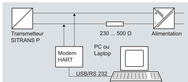
Communication HART entre le PC et le transmetteur de pression
